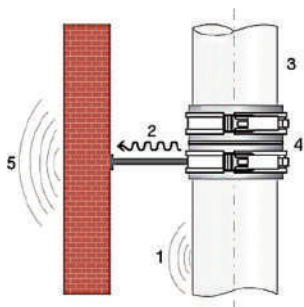
1. Suono di tipo aereo ridotto. - 2. Suono di tipo strutturale ridotto. - 3. Tubo insonorizzato SILENZIO PLUS. - 4. Tecnica di fissaggio corretta. - 5. Insonorizzazione ridotta
